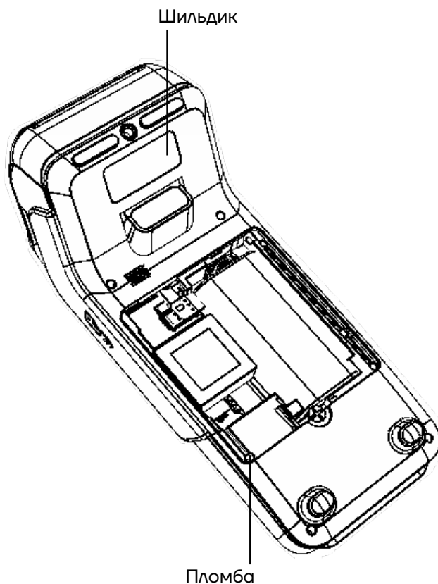
Рисунок 1. Расположение маркировки на корпусе ККТ (крышка АКБ не показана)
