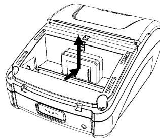
Рисунок 4. Место приложения усилий при извлечении ФН
