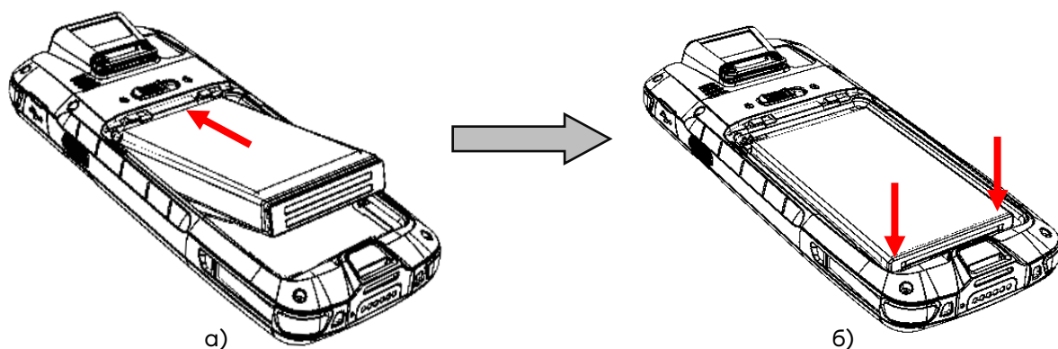
Рисунок 7. Установка АКБ:
